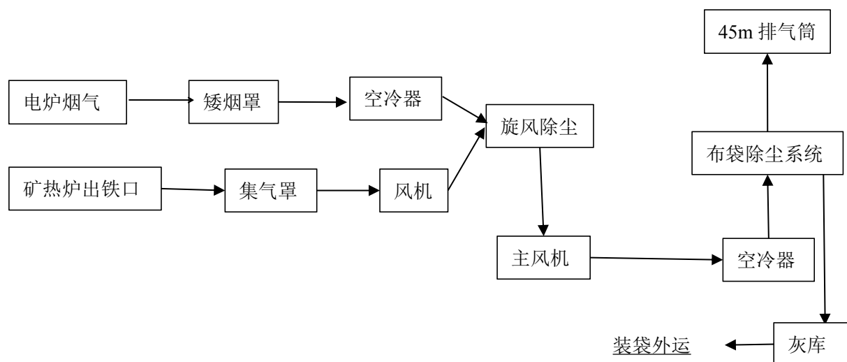
图 4-1 项目运营期废气产生源、废气流向及治理流程
