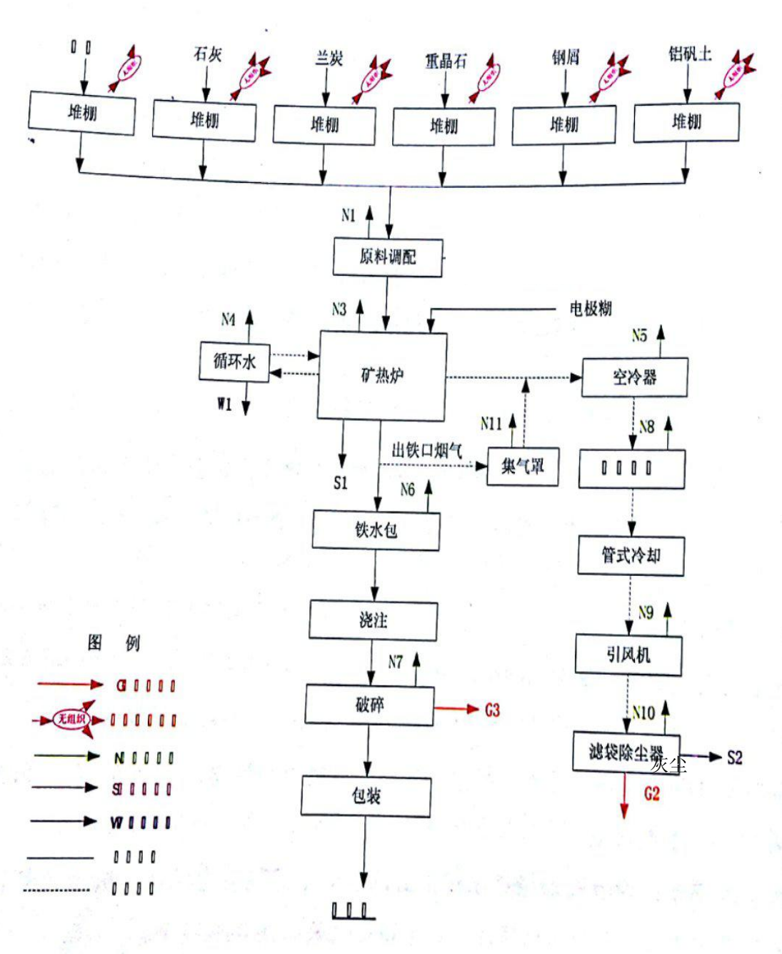
图 3-5 项目生产工艺流程及产污节点图
